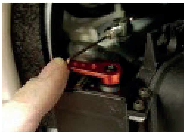
Fig. 3: Chokespjeld åpnet
